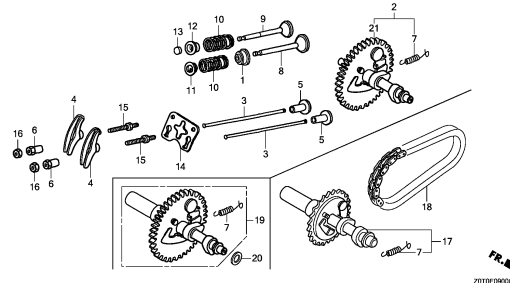
カムシャフト
