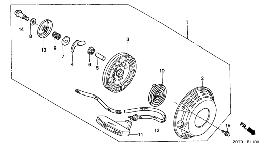
リコイルスターター (1)
