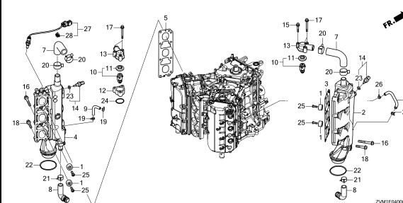
オイルパン(2)
