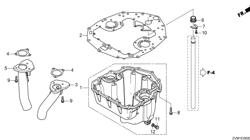
オイルパン(1)
