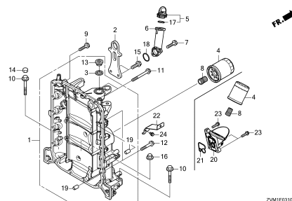
オイルパン(1)
