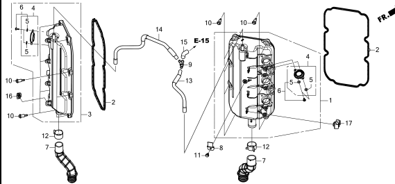
シリンダーヘッドカバー(2)
