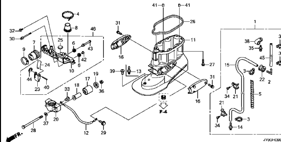
ウォーターポンプ/バーチカルシャフト
