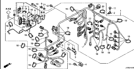
メインワイヤーハーネス
