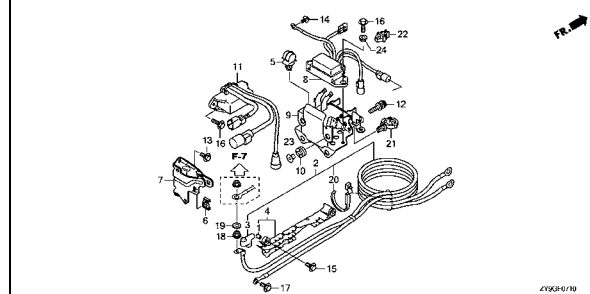
スターターケーブル
