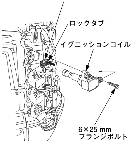
イグニッションコイルカプラー
