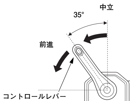
トップマウントリモートコントロール：
