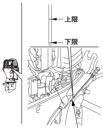
オイルレベルゲージ (検油棒)
