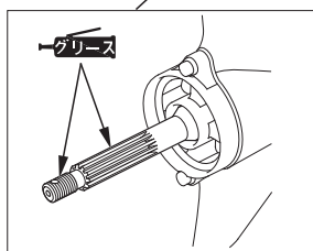
プロペラシャフト
