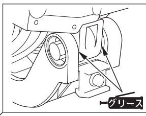
チルトブラケット
