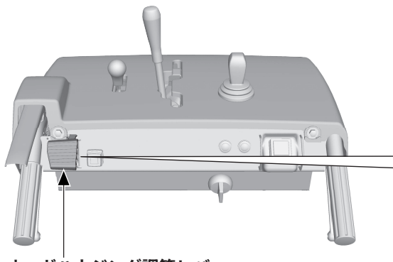
オーガハウジング調節レバー
