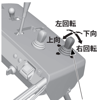
投雪方向調節スイッチ
