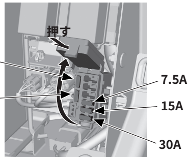
ヒューズボックス
