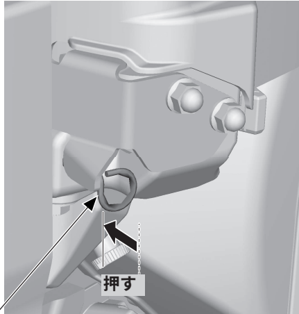
マニュアルスタートレバー
