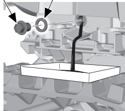
シーリングワッシャー（交換）
