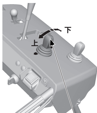
オーガハウジング調節スイッチ
