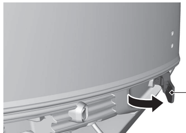
エンジンカバー固定レバー（左右両側）
