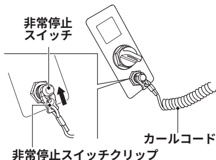
コントロールパネル
