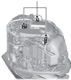
エンジンハンガー
