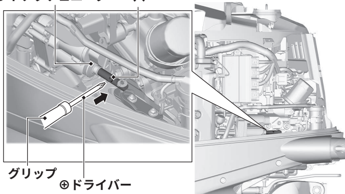
シフトアクチュエーター 穴
