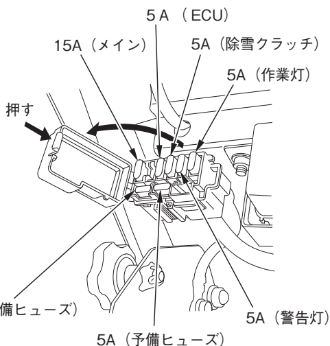
ヒューズボックス
