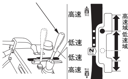
前後進速度調節レバー
