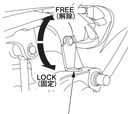
チルトロックレバー
