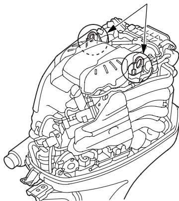
エンジンハンガー
