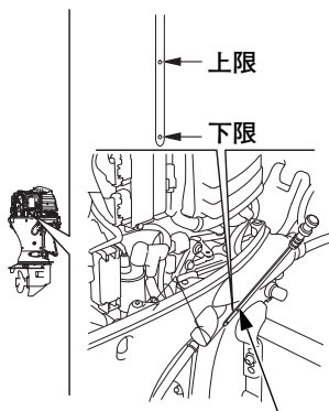
オイルレベルゲージ（検油棒）
