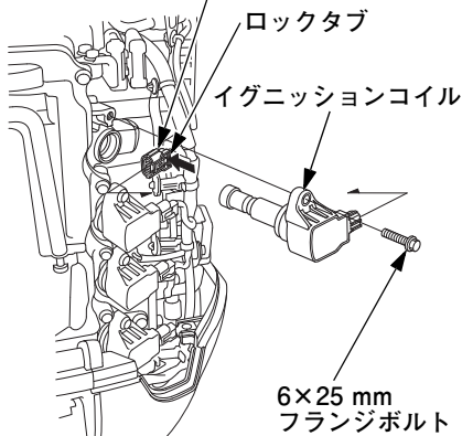
イグニッションコイルカプラー
