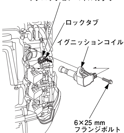
イグニッションコイルカプラー
