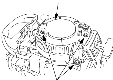
6 mm ボルト
