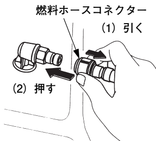
（タンク側）
