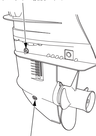
ギアオイルドレンスクリュー
