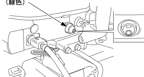
エンジン オイル油圧表示灯 (緑色)
