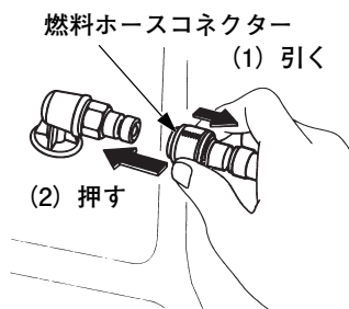
（外部燃料タンク側）
