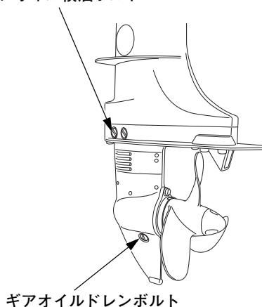
ギアオイル検油ボルト
