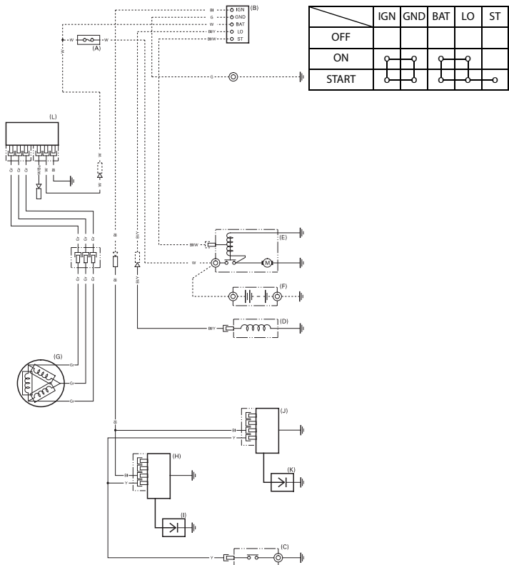
Tipo con bobina de carga de 26 A y sin caja de control
