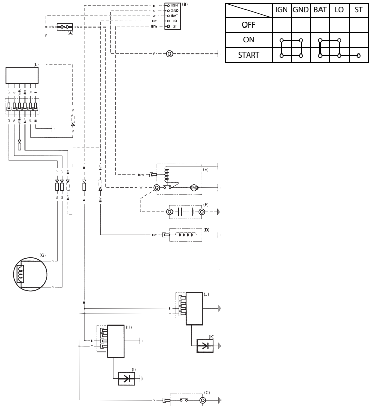
Tipo con bobina de carga de 17 A y sin caja de control
