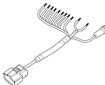
Molex MX150 12-polig Steckverbinder, Kabelansicht und Kabelbaum (mitgeliefert)
