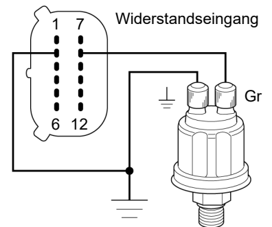
Drucksensor mit isolierter Masse an Widerstandseingang 8 angeschlossen
