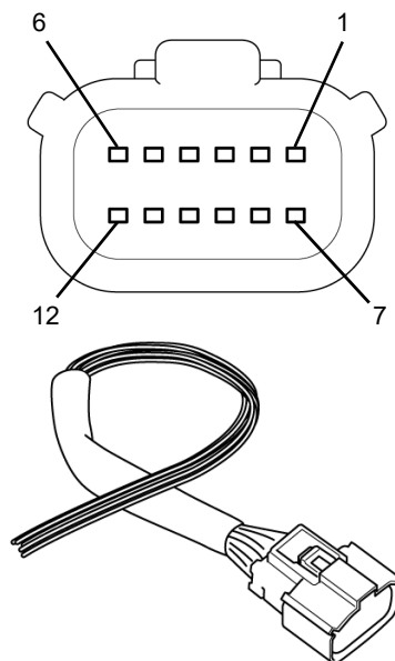
Conector Molex MX150 de 12 polos, vista del cable y mazo de cables (componentes opcionales fabricados por Veratron)
