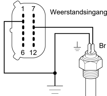
Temperatuursensor met geïsoleerde aarde aangesloten op weerstandsingang 9
