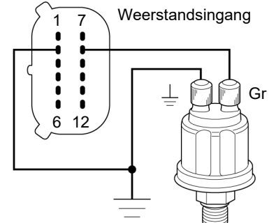
Druksensor met geïsoleerde aarde aangesloten op weerstandsingang 8
