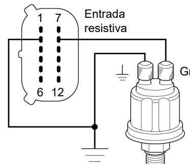
Sensor de presión con tierra aislada conectado a la entrada resistiva 8
