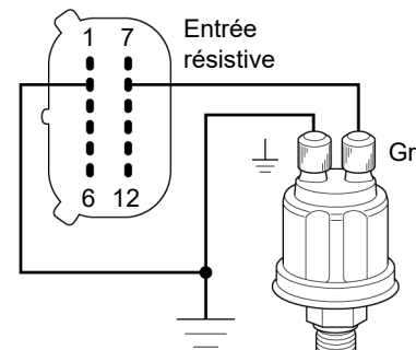
Capteur de pression avec masse isolée raccordée à l'entrée résistive 8
