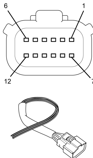
Molex MX150 12-polige connector, kabelzicht en kabelboom (optionele componenten gemaakt door Veratron)
