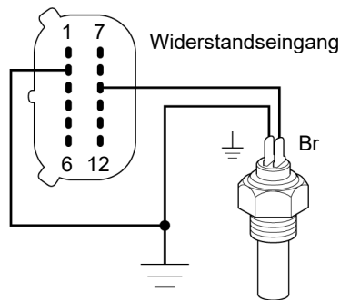
Temperatursensor mit isolierter Masse an Widerstandseingang 9 angeschlossen
