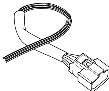
Molex MX150 12-poliger Steckverbinder, Kabelansicht und Kabelbaum (Von Veratron hergestellte optionale Komponenten)
