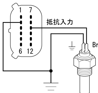
抵抗入力 (9) に接続された 絶縁アース付き温度センサー
