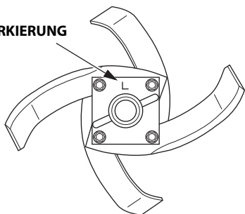
LINKER ÄUSSERER ZINKEN (Von innerer Zinkenseite aus gesehen)
