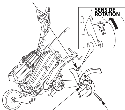
PIECE ROTATIVE INTERNE GAUCHE
