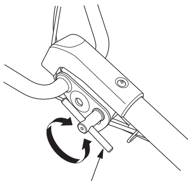
LENKER-HÖHEREINSTELLHEBEL
