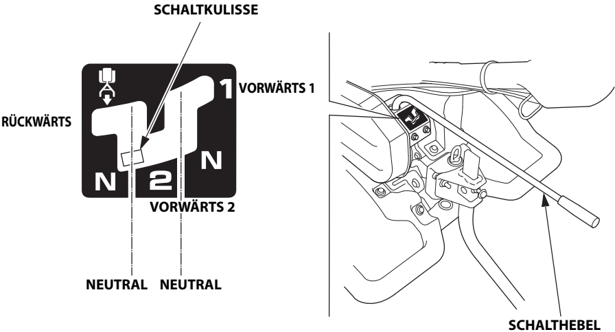
Gangwahltabelle (bei einer Motordrehzahl von 3.600 min -1 )
