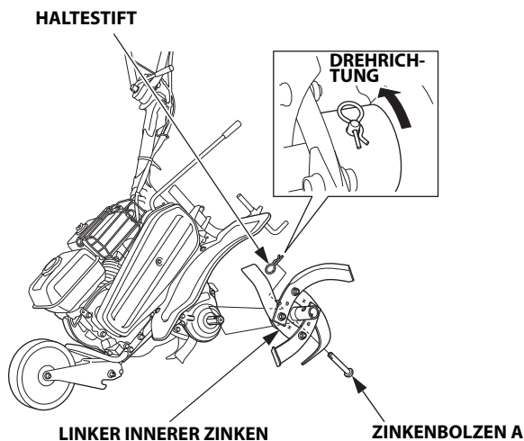
ZINKENBOLZEN A (LANG)
