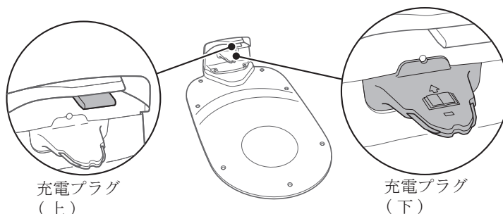
充電プラグ (下) の金属接点
