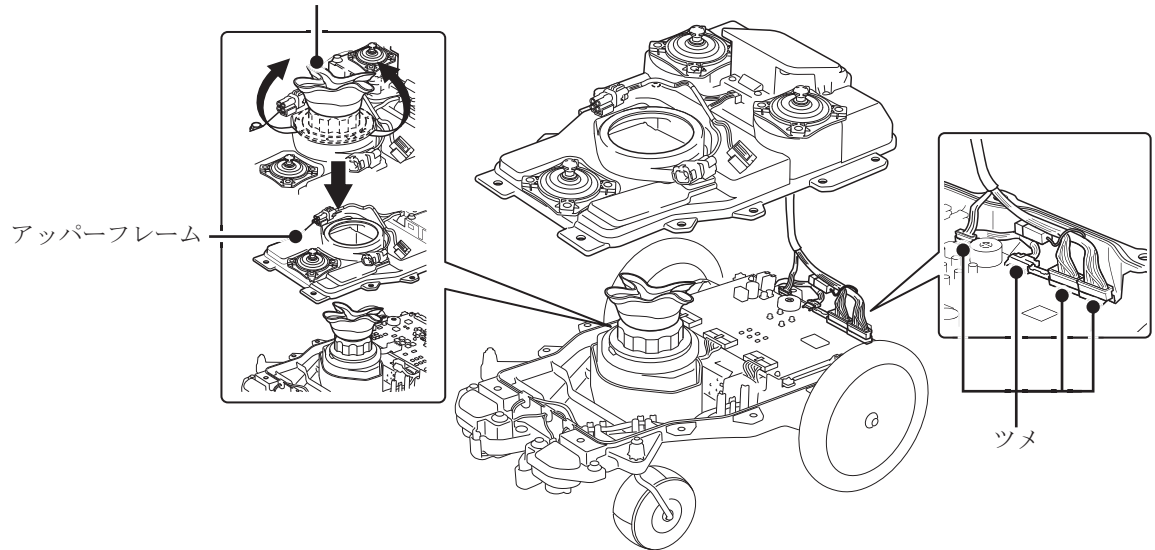
刈高調整ダイアルのキャップ
