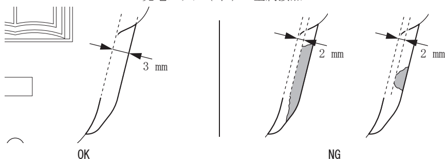
充電プラグ (下) の金属接点
