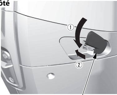
LEVIER DE VERROUILLAGE DU CAPOT MOTEUR (de chaque côté)
