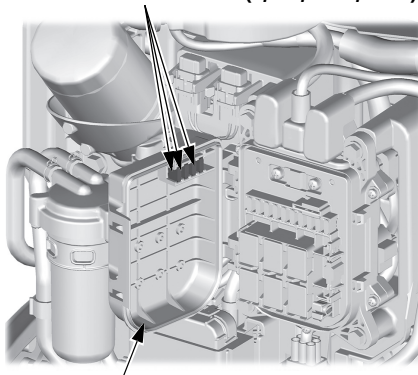
COUVERCLE DU BOÎTIER DE RACCORDEMENT
