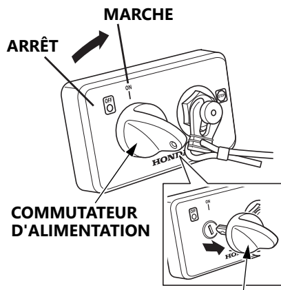
CLÉ DU COMMUTATEUR D'ALIMENTATION
