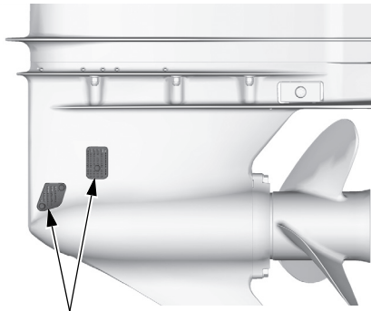
ORIFICE D'ADMISSION DE L'EAU DE REFROIDISSEMENT (de chaque côté)
