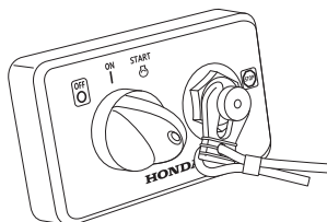
CLÉ NORMALE SANS COMMUTATEUR DE DÉMARRAGE/ARRÊT
