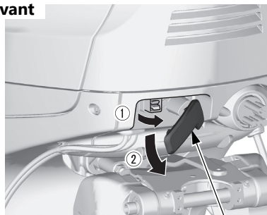
LEVIER DE VERROUILLAGE DU CAPOT MOTEUR
