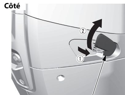
LEVIER DE VERROUILLAGE DU CAPOT MOTEUR (de chaque côté)
