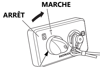
COMMUTATEUR D'ALIMENTATION
