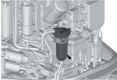
FILTRE À CARBURANT AVEC SÉPARATEUR D'EAU (CÔTÉ BASSE PRESSION)
