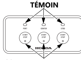
COMMUTATEUR DÉMARRAGE/ARRÊT
