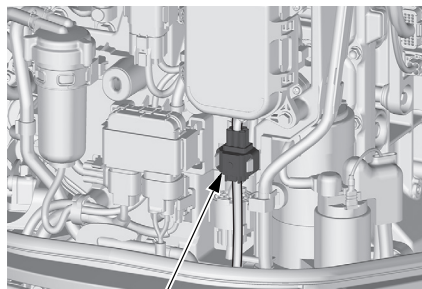
CONNECTEUR D'INTERFACE NMEA
