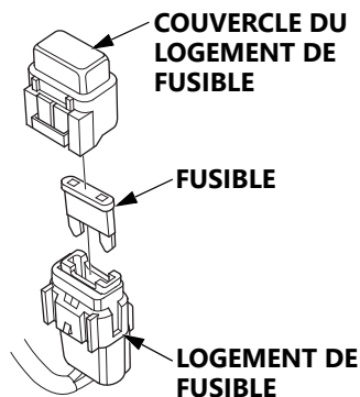
FUSIBLES DE RECHANGE (3 A, 7,5 A)
