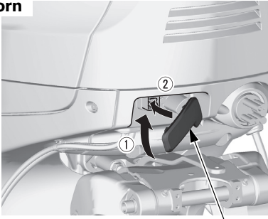
MOTORABDECKUNGSRASTHEBEL
