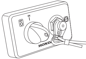
NORMALER SCHLÜSSEL MIT START/STOPP-SCHALTER
