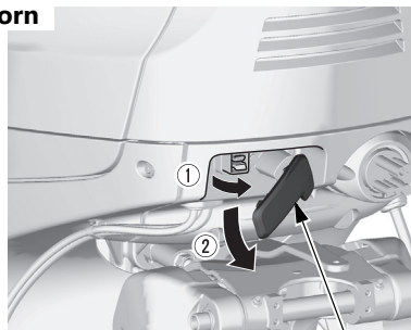
MOTORABDECKUNGSRASTHEBEL
