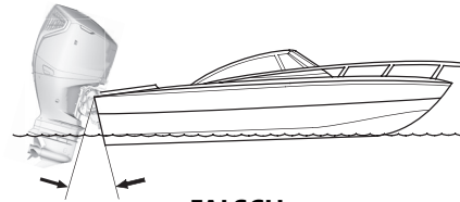
FALSCH BOOT WIRD HECKLASTIG
