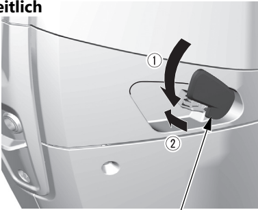
MOTORABDECKUNGSRASTHEBEL (auf jeder Seite)
