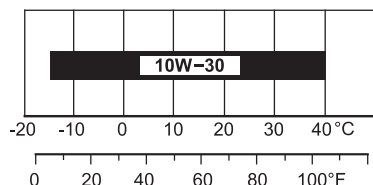
UMGEBUNGSTEMPERATUR
