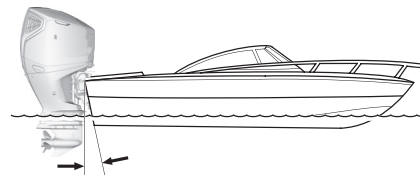
RICHTIG BOOT LIEGT RICHTIG IM WASSER, BESTE KRAFTAUSNUTZUNG
