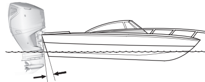
FALSCH BOOT WIRD BUGLASTIG
