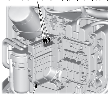
VERTEILERKASTENDECKEL
