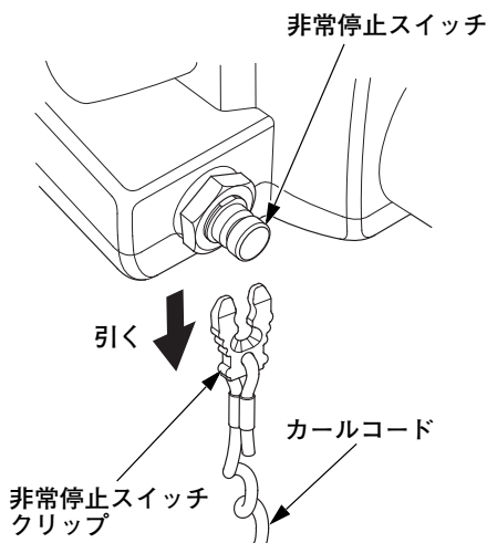
〔ティラーハンドル仕様〕
