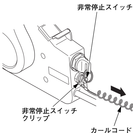
〔リモートコントロール仕様〕 サイドマウントリモートコントロール：
