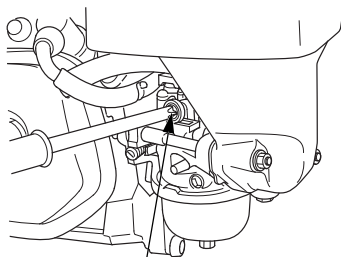
VITE DI ARRESTO VALVOLA A FARFALLA
