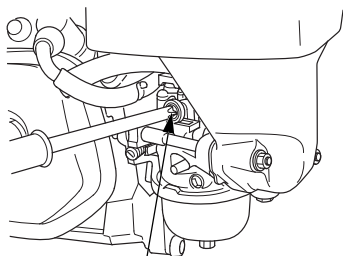
DROSSELANSCHLAGSCHRAUBE
