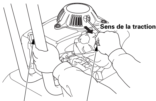
(COTE EQUIPEMENT) POIGNEE DE LANCEMENT
