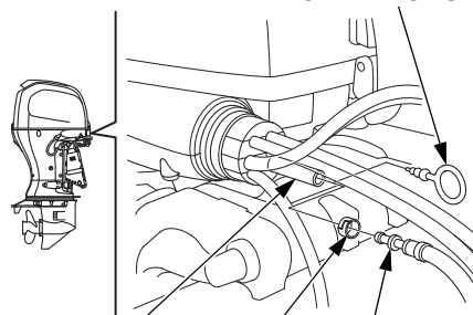
RACCORDO CONDOTTO CARBURANTE
