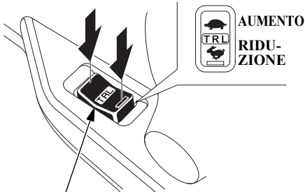
INTERRUTTORE DI CONTROLLO TRL (regime di traina)
