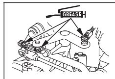
BRACCIO/ARTICOLAZIONE/ PERNO/PIASTRA DELL'ACCELERATORE
