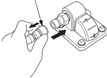
CONNETTORE TUBO CARBURANTE (al serbatoio carburante)
