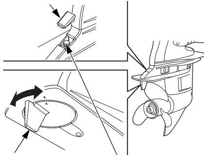
PINNA DIREZIONALE
