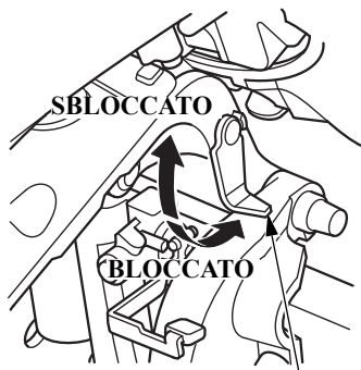
LEVA PER IL BLOCCAGGIO DEL SOLLEVAMENTO
