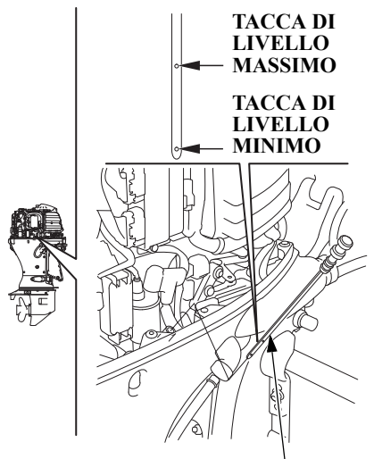
ASTINA DI MISURAZIONE LIVELLO OLIO
