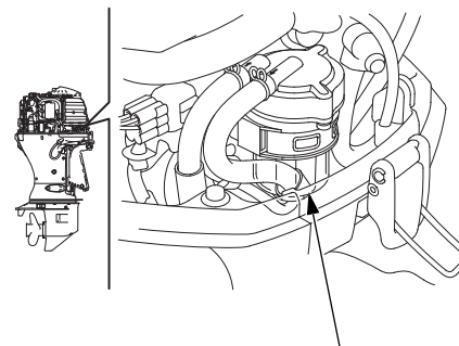
SEPARATORE D'ACQUA
