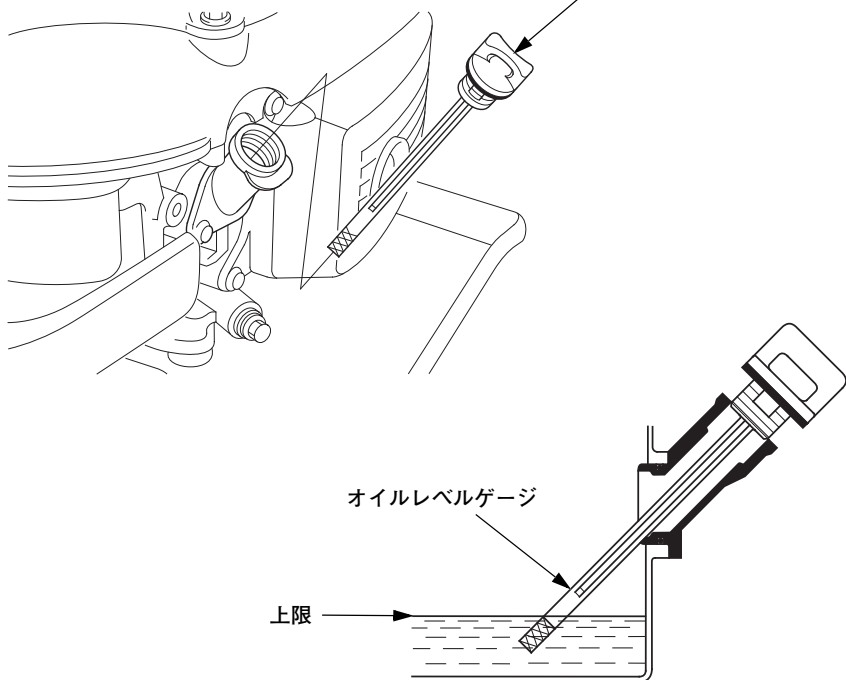
オイル給油キャップ／ オイルレベルゲージ
