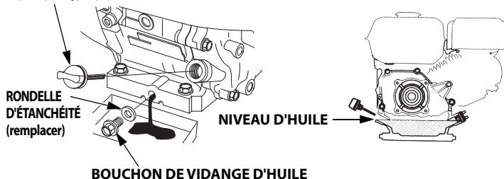
BOUCHON DE REMPLISSAGE D'HUILE/JAUGE
