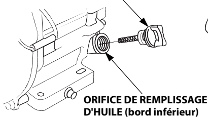
BOUCHON DE REMPLISSAGE D'HUILE/JAUGE
